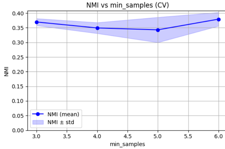
الشكل 49: أثر معامل حجم العينات على النتائج.
