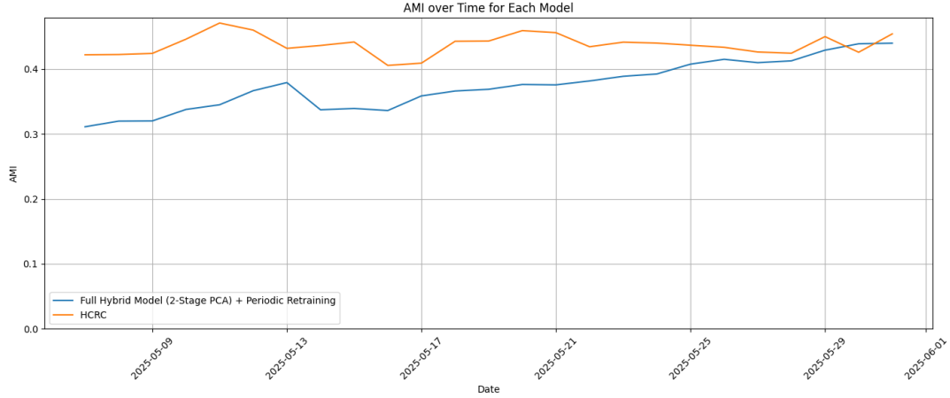
الشكل 94: مقارنة النموذج المقترح مع النموذج المرجعي وفق معيار AMI.
