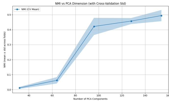
الشكل 45: أثر عدد الأبعاد على نتائج العقدة.
