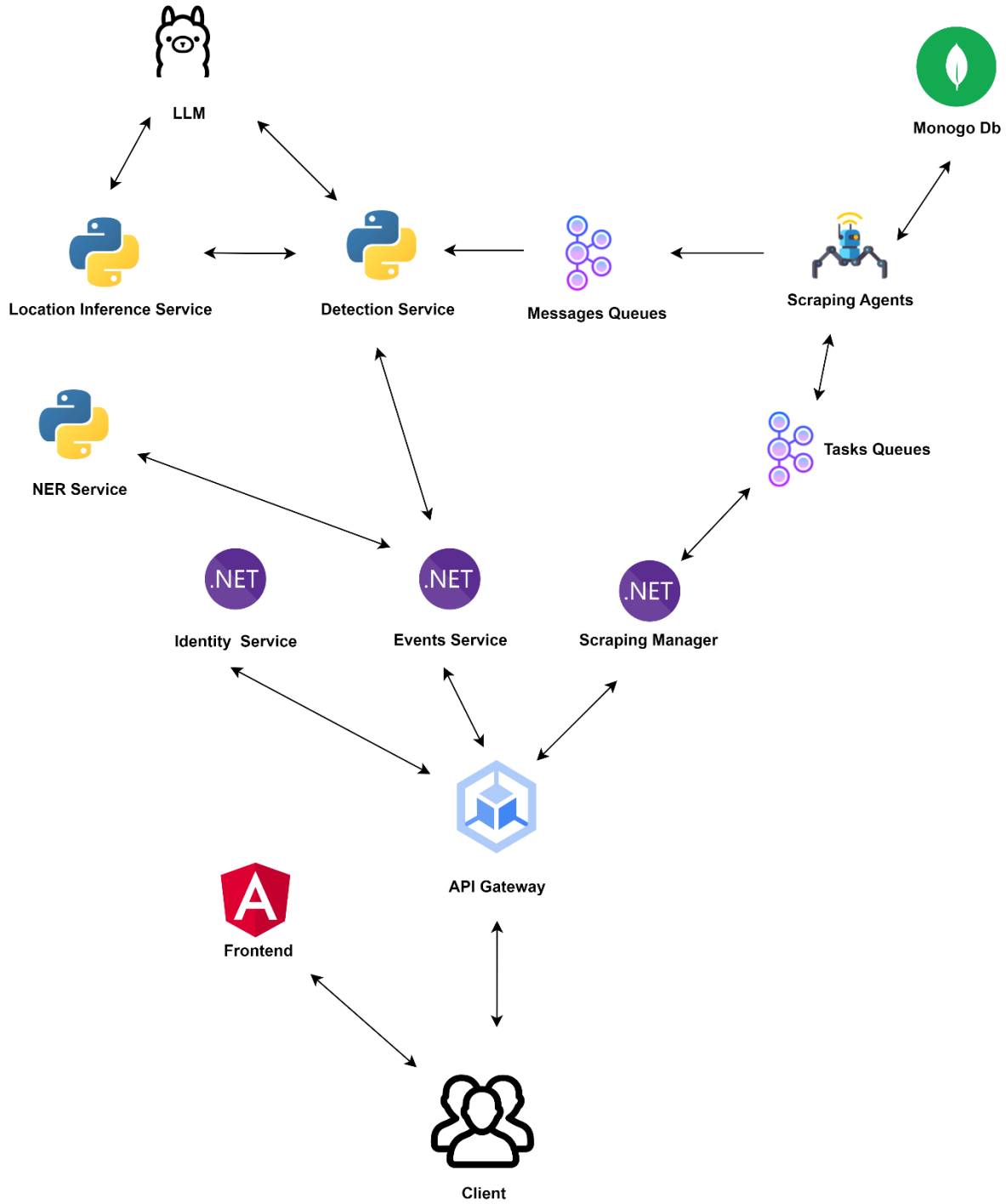
الشكل 91: مخطط النظام التنفيذي.
