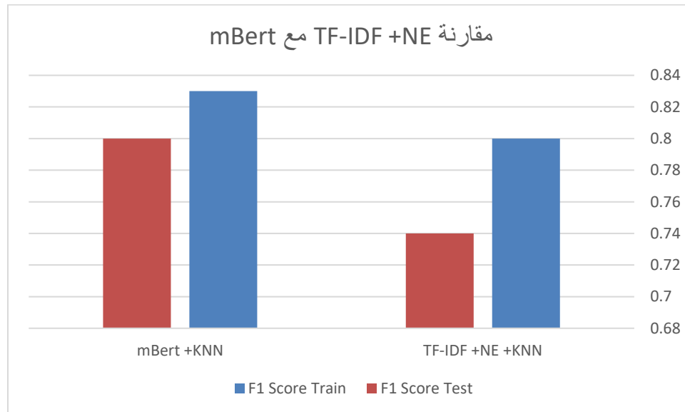
الشكل 39: مقارنة TF-IDF +NE مع mBert.
