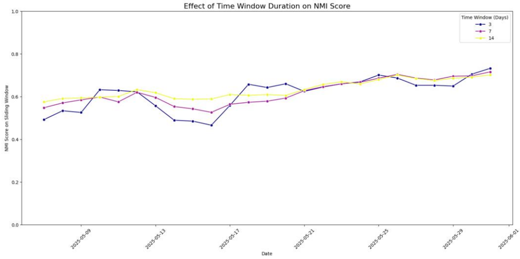
الشكل 69: أثر حجم النافذة الزمنية على نتائج العقدة.
