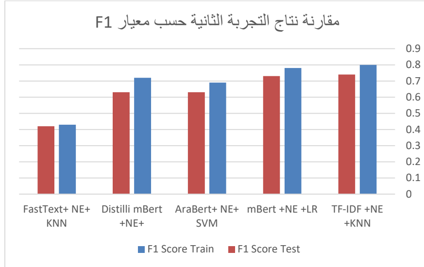
الشكل 38: مخطط مقارنة نتائج التجربة الثانية حسب معيار F1.
