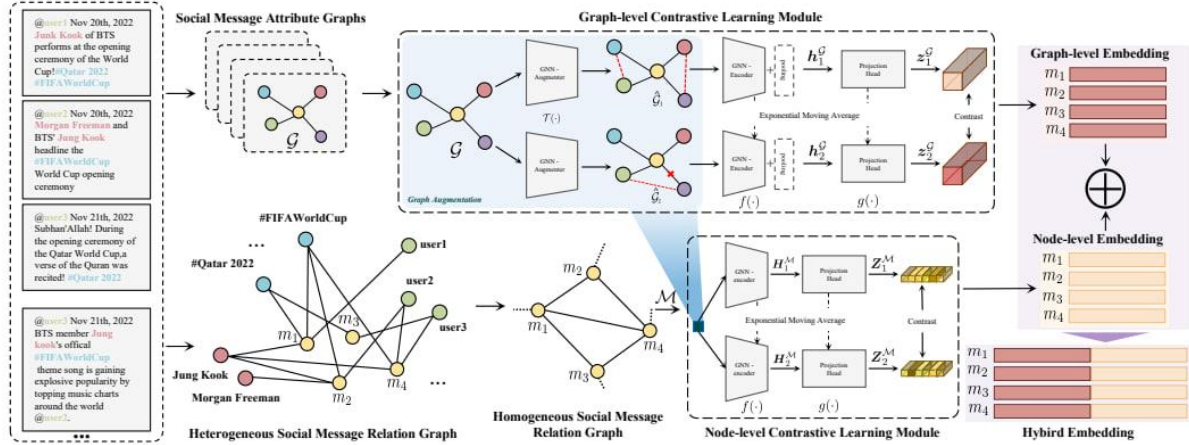
الشكل 9: تفاصيل بناء البيان والتعلم المقارن في النموذج HCRC.
