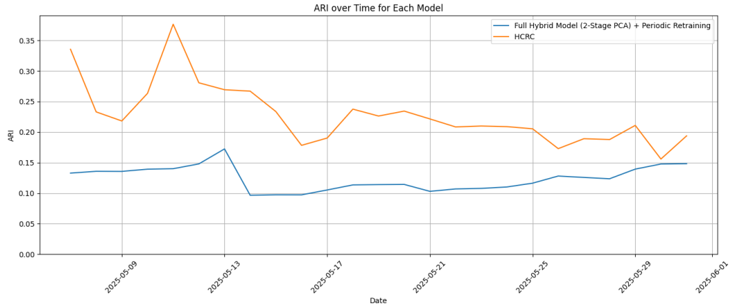
الشكل 67: مقارنة النموذج المقترح مع النموذج المرجعي وفق معيار ARI.
